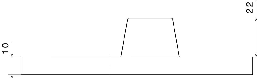
Vue de gauche Echelle : 1:1
